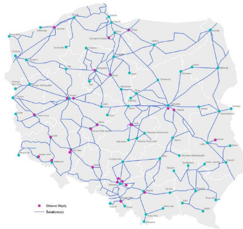
Aktualny zasięg światłowodowej sieci szkieletowej Netii
